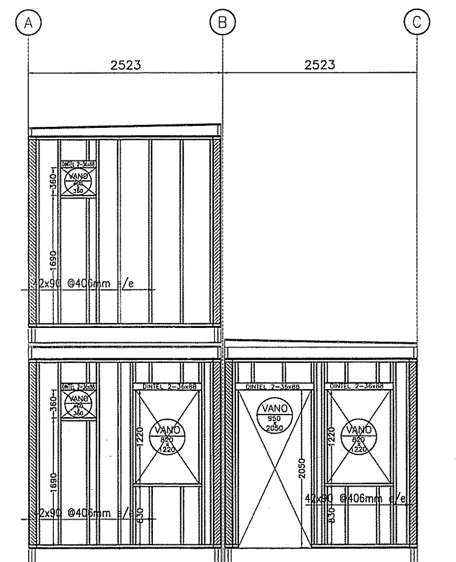
ELEVACION ESTRUCTURA EJE 1; CARA EXTERIOR CON OSB e=9.5mm esc:1/50
