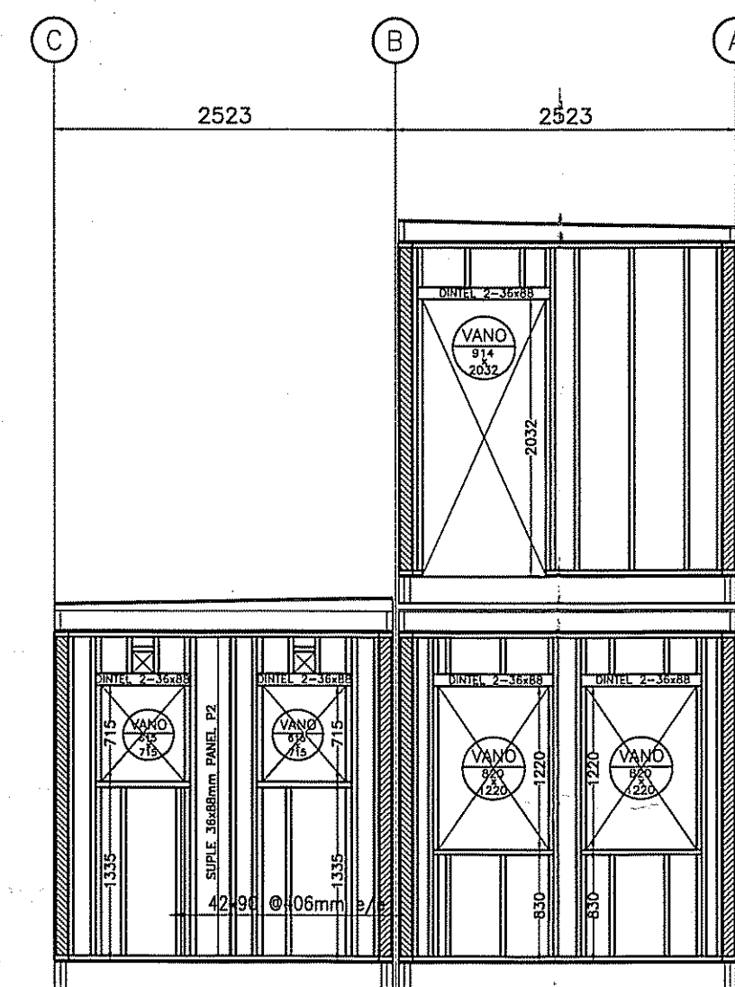
ELEVACION ESTRUCTURA EJE 3-2; CARA EXTERIOR CON OSB e=9.5mm esc:1/50
