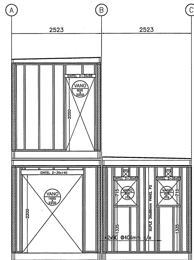
ELEVACION ESTRUCTURA EJE 2; CARA EXTERIOR CON OSB e=9.5mm esc:1/50
