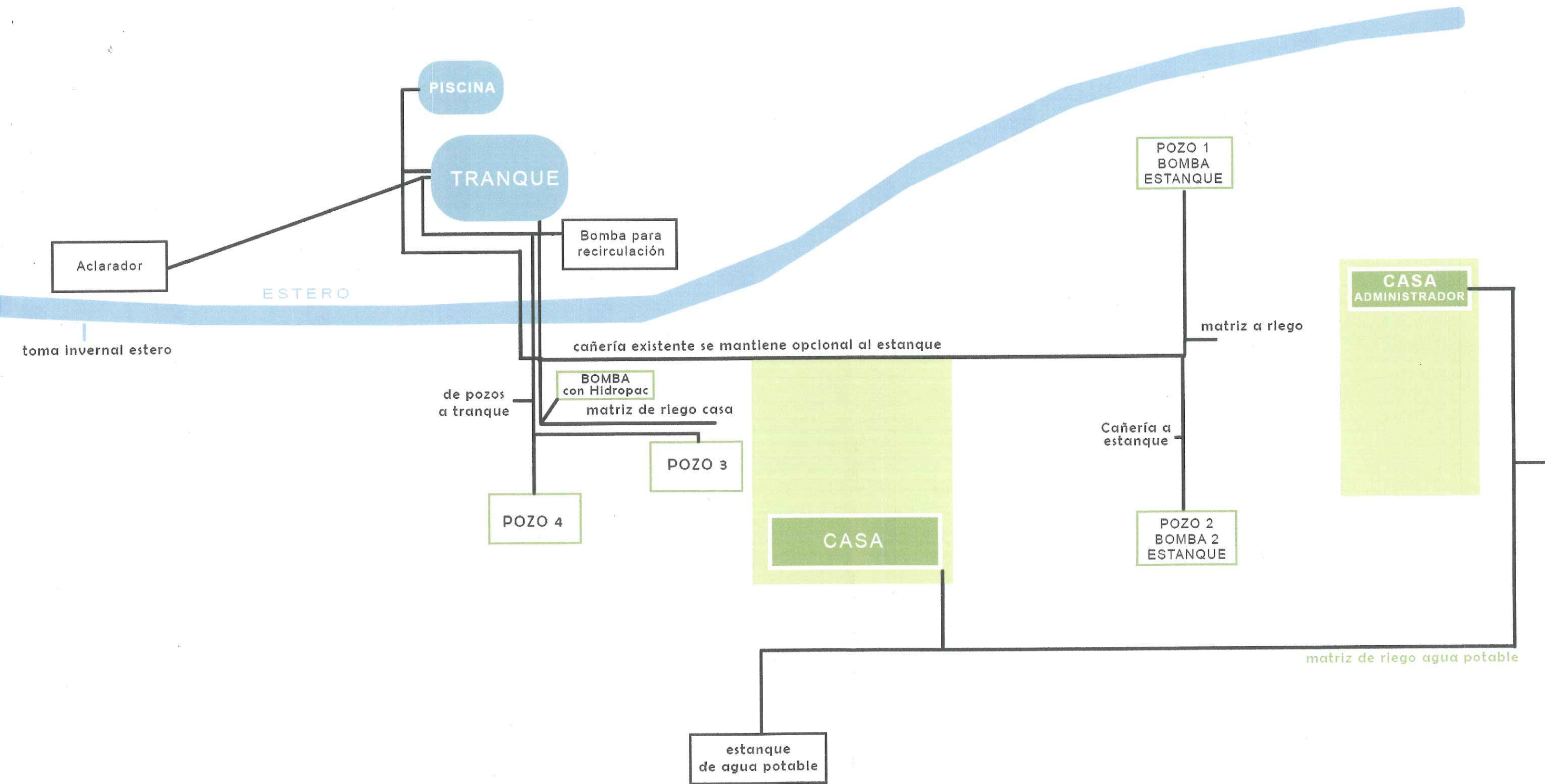
ESQUEMA DE AGUAS FUNDO SANTA SOFIA
